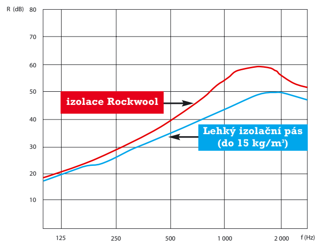
Porovnání vzduchové neprůzvučnosti dvou různých izolačních materiálů (obr. 36)
