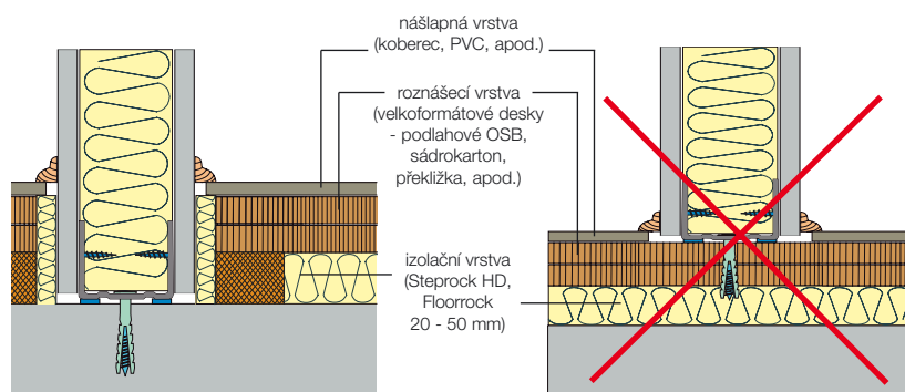
Správné napojení příčky a plovoucí podlahy na nosnou konstrukci - svislý řez (obr. 22)
