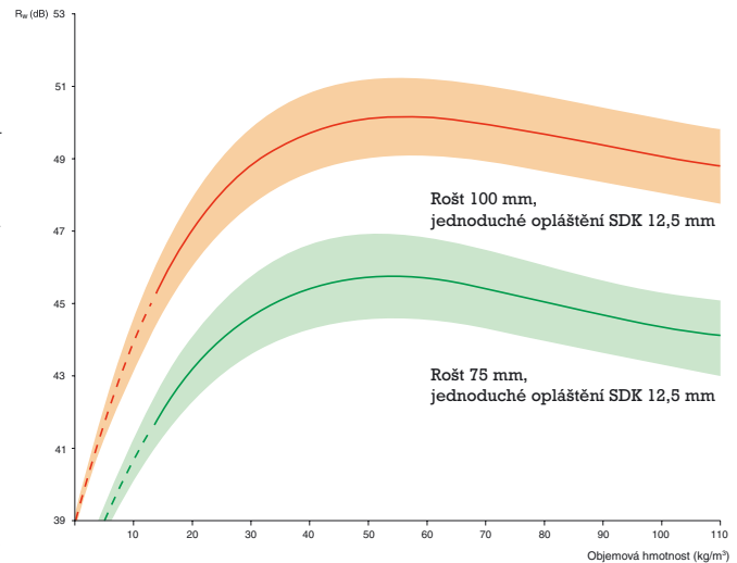
Závislost vzduchové neprůzvučnosti R_w na objemové hmotnosti použité izolace (obr. 34)
