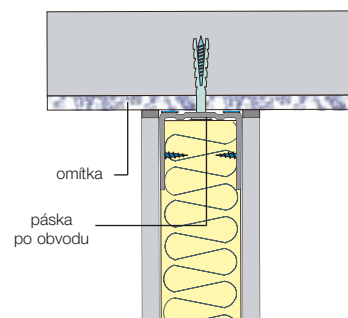
Napojení příčky na strop - svislý řez (obr. 24)
